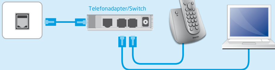
Bredbandsuttag
