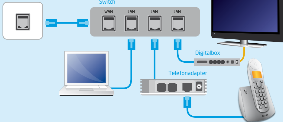
Bredbandsuttag
